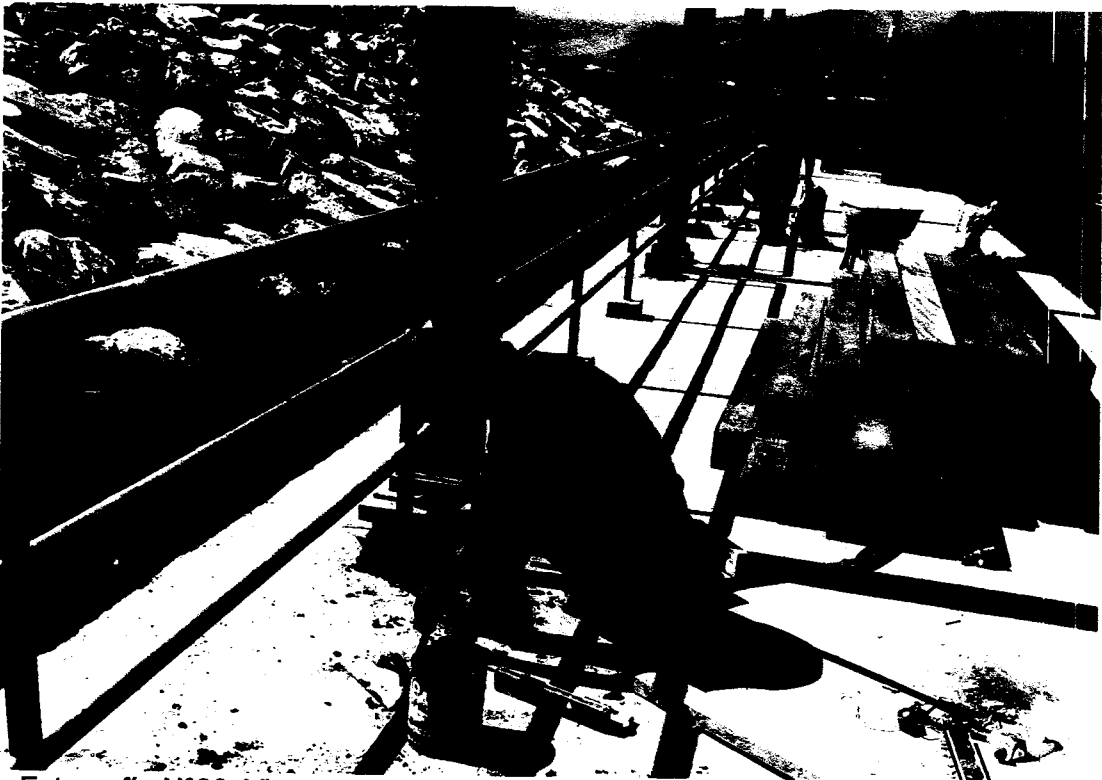
Fotografía N°06: Vista de resane de dados de concreto para barandas en muelle espigón.
